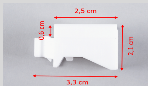
Quote e ingombro del supporto
